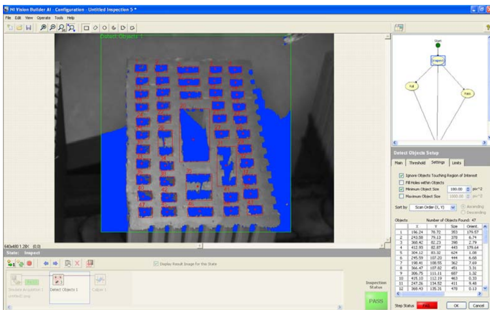
Bild: Visuelle Qualitätskontrolle an einem Ziegelstein
